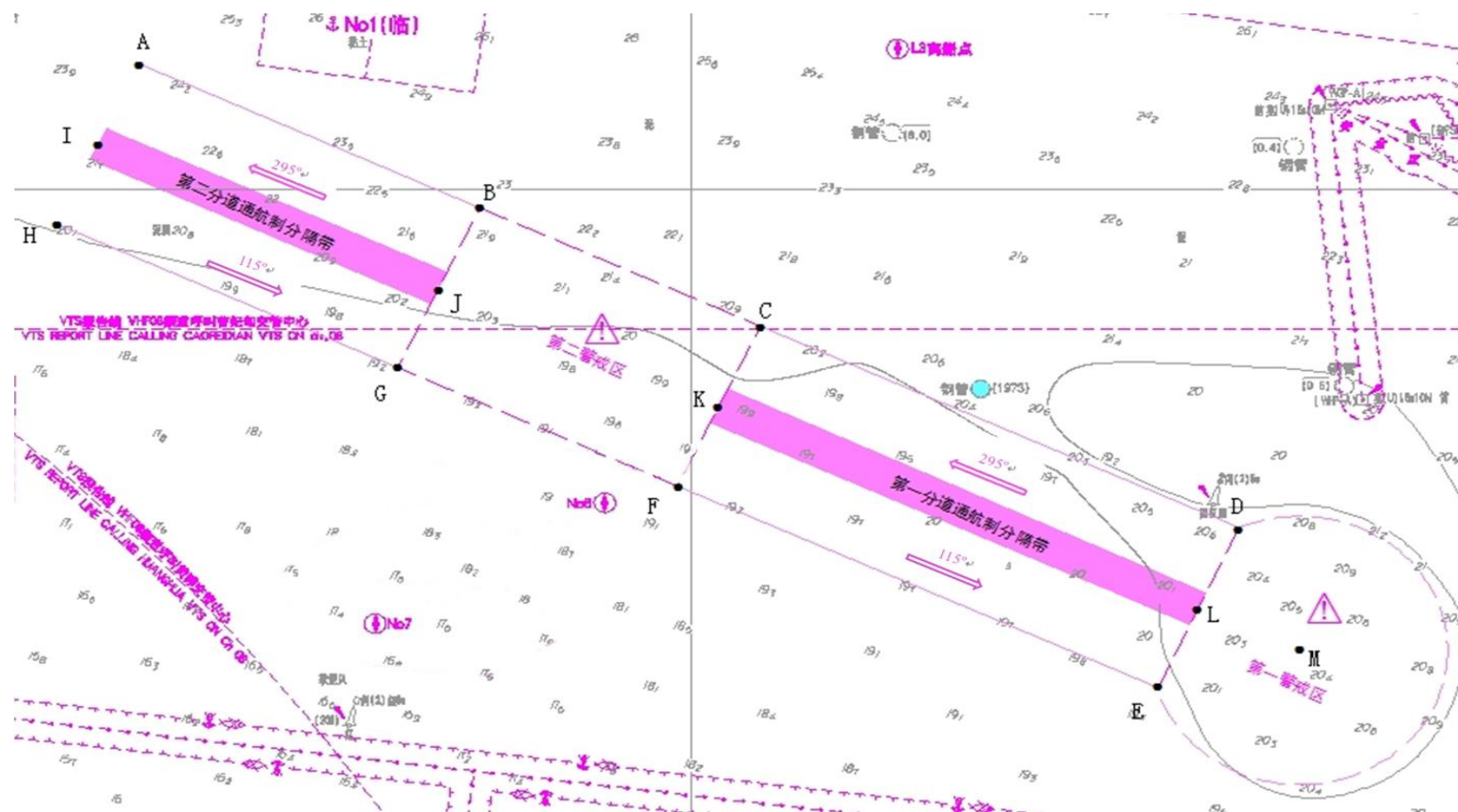
渤海湾中部水域船舶定线制（试行）示意图
